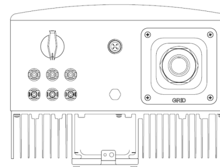
Рисунок 1.2 – Вид снизу
